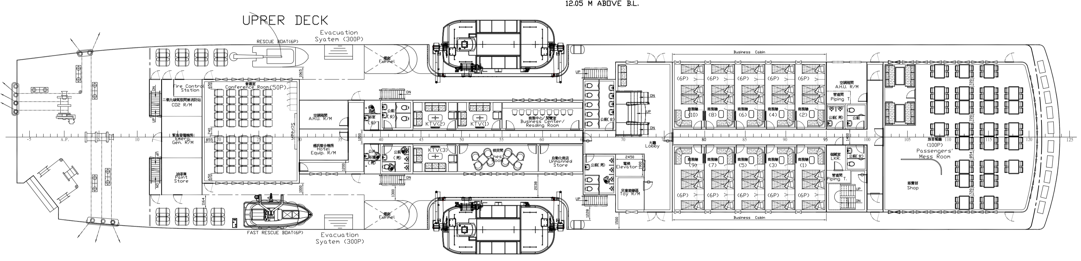
上層甲板 UPPER DECK 12.85 M ABOVE BL.
