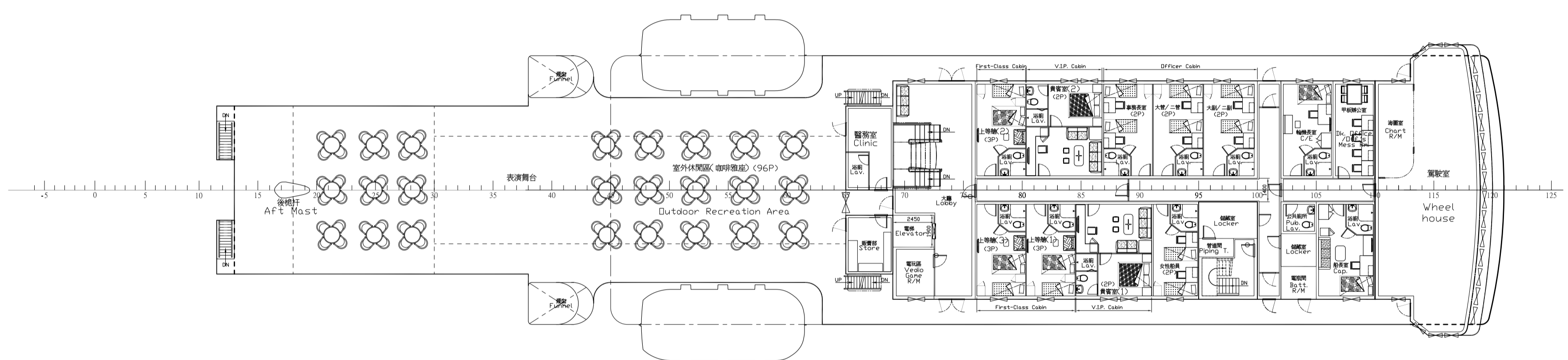
航海船橋甲板 NAV. BRIDGE DECK 14.60 M ABOVE BL.
