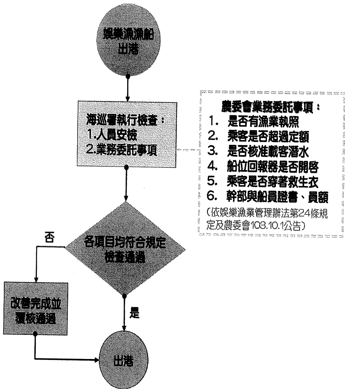
圖 4 娛樂漁業漁船出港前檢查流程
