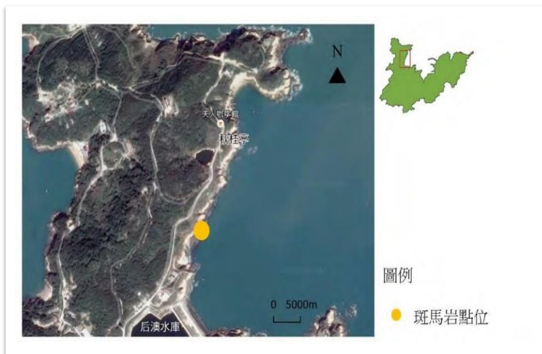
圖2 南竿斑馬岩位置圖
